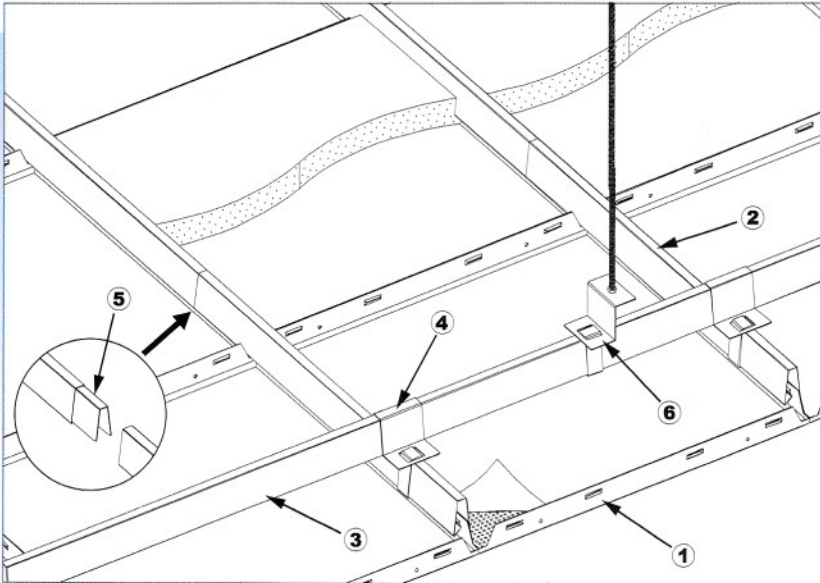
Suspension Drawing : 102 Clip-in Ceiling System 吊掛示意圖 : 102暗架天花系統
