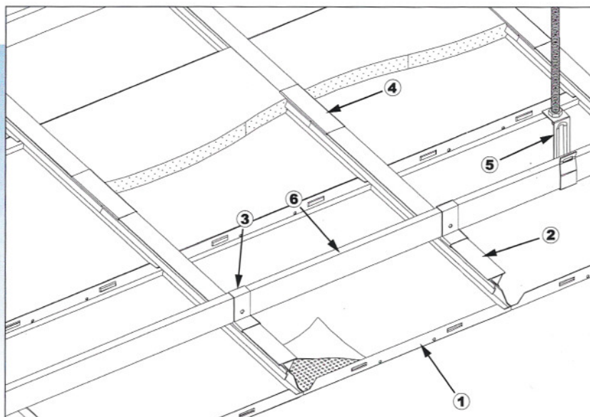
Suspension Drawing : 101 Clip-in Ceiling System 吊掛示意圖：101 暗架天花系統
