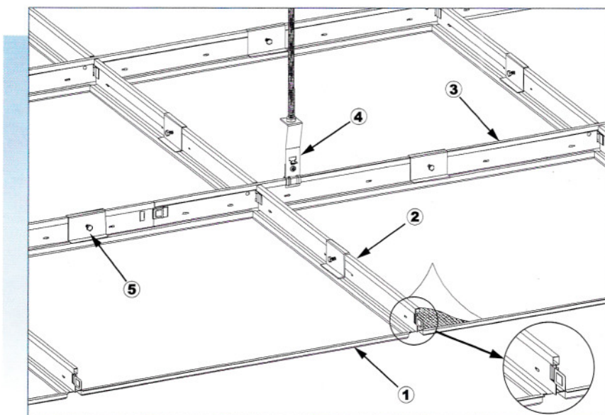
Suspension Drawing : 201 Lay-in Ceiling System 吊掛示意圖：201 明架跌級天花系統
