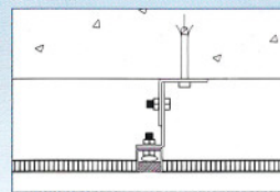
Horizontal Section 水平切面圖
