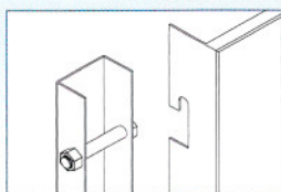
Installation Details 組裝詳細圖
