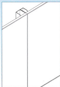
Cladding Installation 牆身板組裝完成圖
