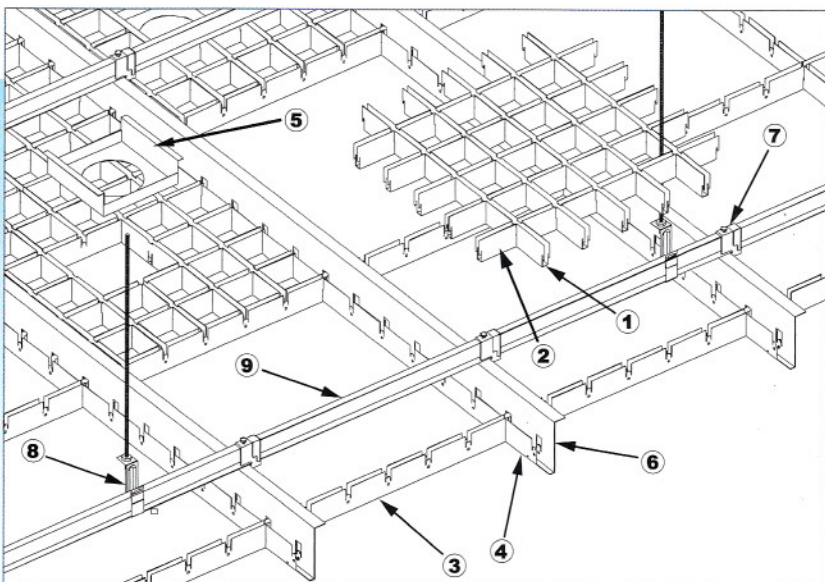
Suspension Drawing : 3000 External Cell Ceiling System 吊掛示意圖：3000 室外網格天花系統
