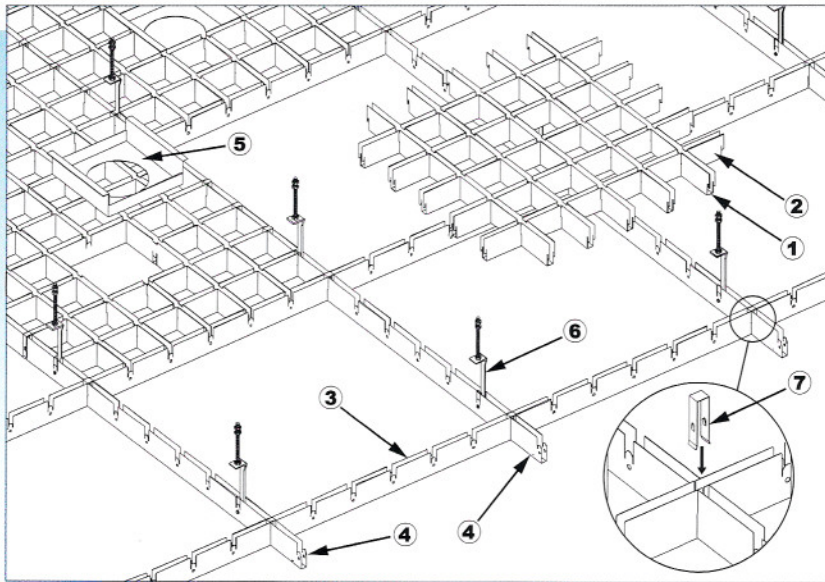
Suspension Drawing : 2000 External Cell Ceiling System 吊掛示意圖：2000 室外網格天花系統
